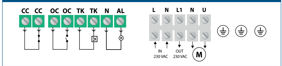
Мал. 3 Схема підключення
