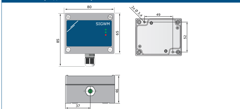
Мал. 1 Розміри для монтажу
