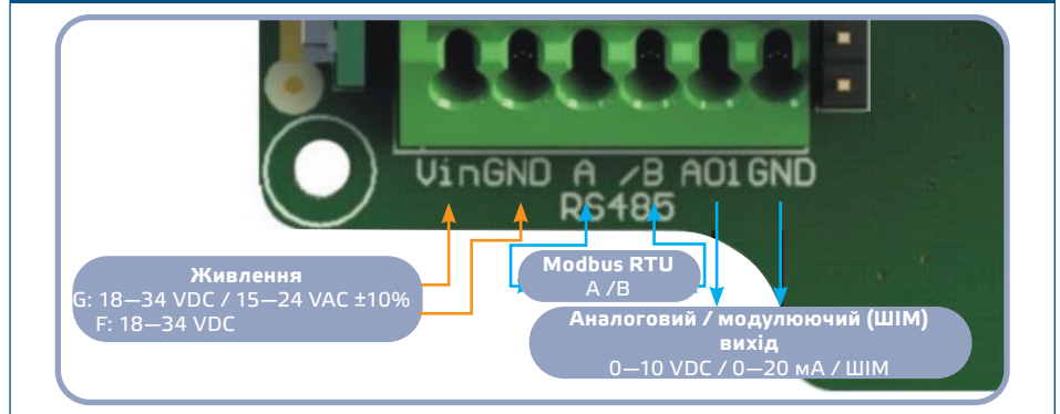
Мал. 3 З'єднання
