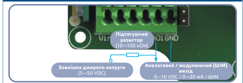
Мал. 5 З'єднання ШІМ (Відкритий колектор)
