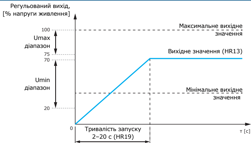
Рис. 4 Плавний запуск
