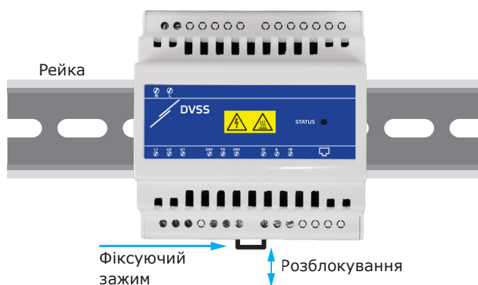
Рис. 2 Монтажне положення
