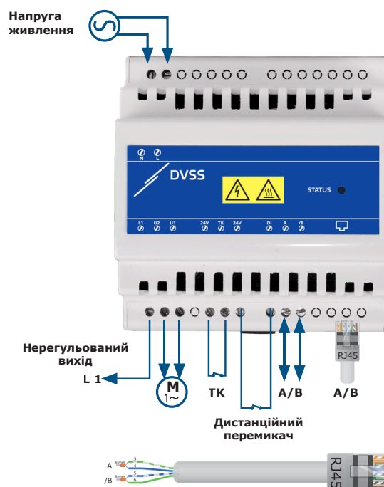
Рис. 3 Схема підключення
