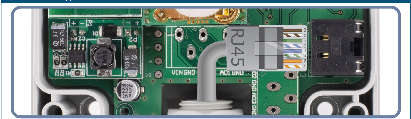
Мал. 4 Схема підключення
