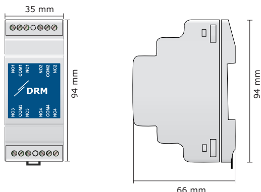
Мал. 1 Монтажні розміри
