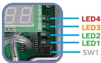
Мал. 8 Калібрування датчика і скидання реєстра Modbus
