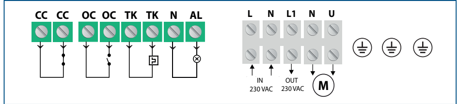
Мал. 3 Схема підключення
