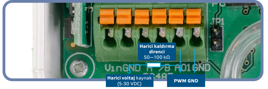
Şek. 6 PWM (Açık kollektör) bağlantısı (JP1 bağlantısı kesildi)
