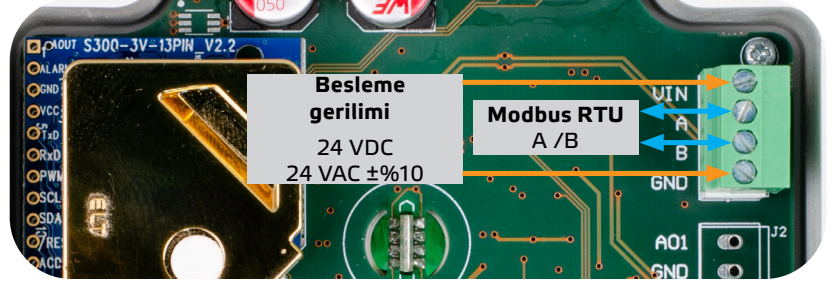
Şek. 3 Kablolama şeması
