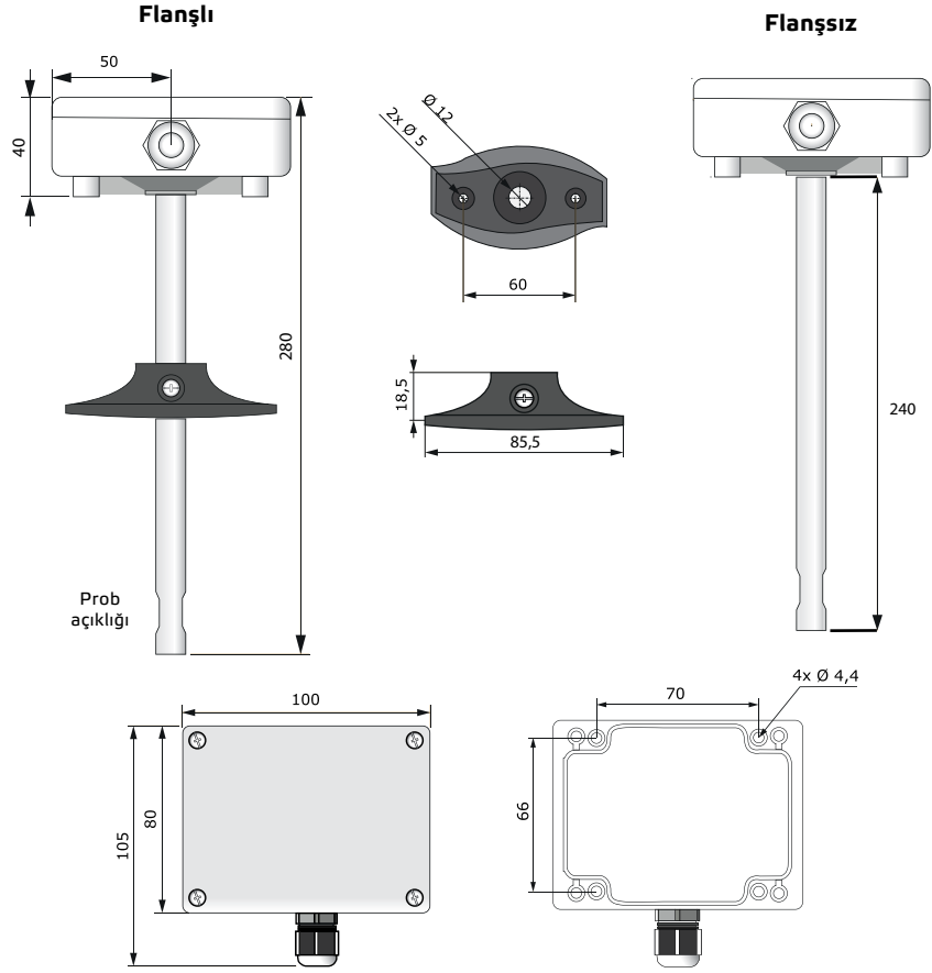
Şek. 1 Montaj boyutları
