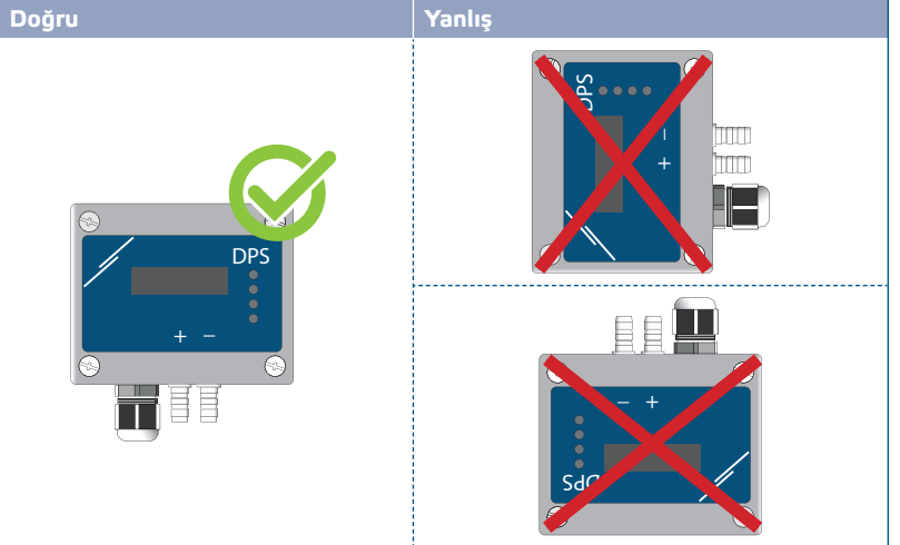
Şek. 2 Montaj konumu
