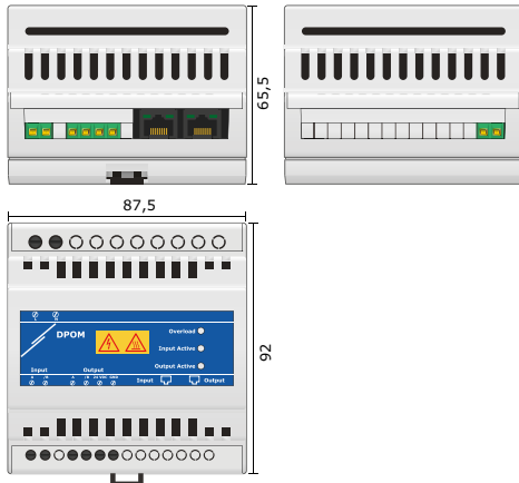
Şek. 1 Montaj boyutları
