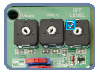
Fig. 7 Trimmer OFF-nivå
