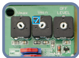
Fig. 6 Min. hastighetstrimmer
