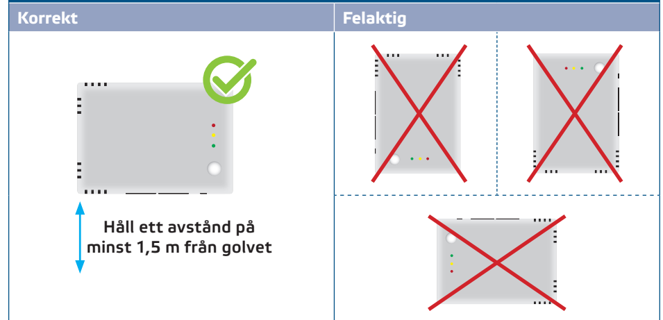
Fig. 3 Monteringsposition
