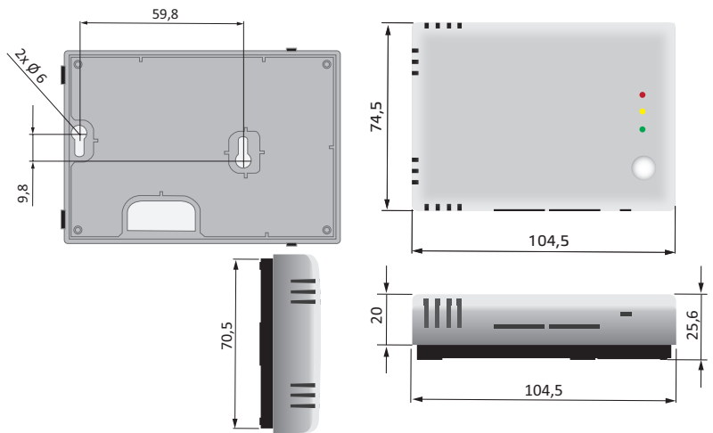
Fig. 2 Monteringsmått
