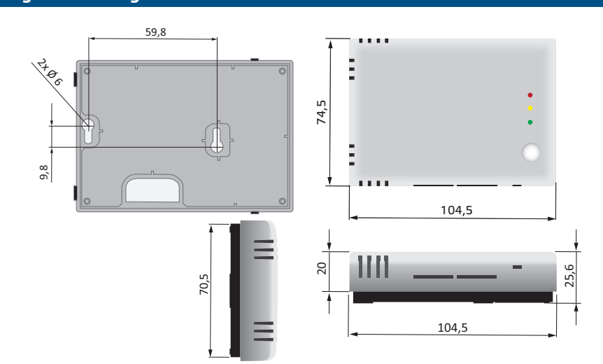
Fig. 2 Monteringsmått
