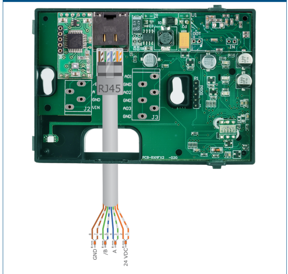
Fig. 4 Koppling
