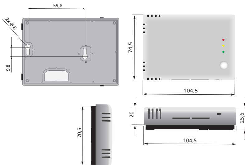
Fig. 2 Monteringsmått
