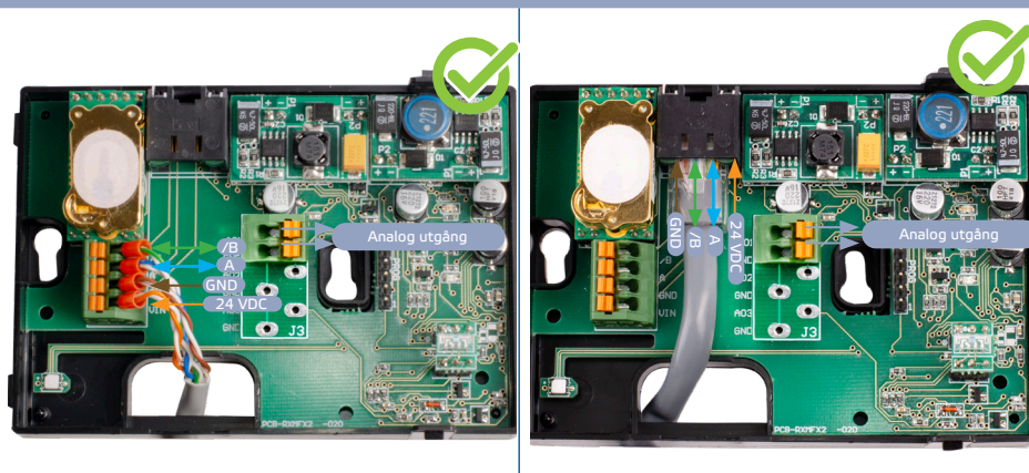
Fig. 4 Koppling och anslutningar
