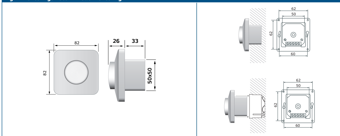
Fig. 2 Monteringsmått – infälld montering
