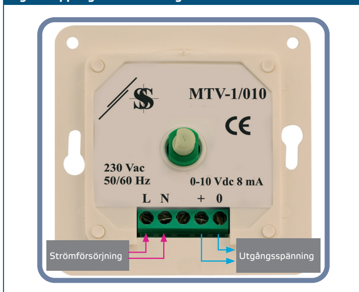
Fig. 1 Koppling och anslutningar
