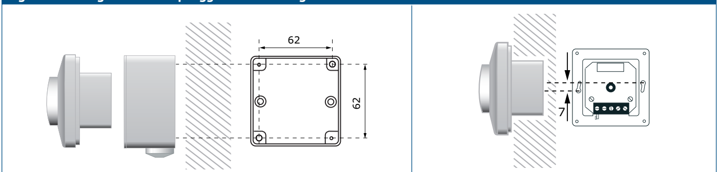
Fig. 3 Monteringsmått - Utanpåliggande montering
