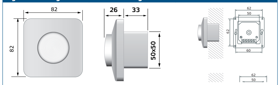
Fig. 2 Monteringsmått - Infälld montering
