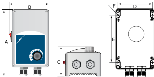
Bild 1 Monteringsmått
