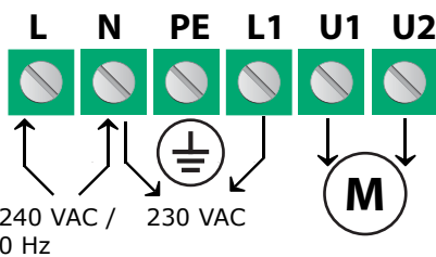
Bild 3 Anslutningar
