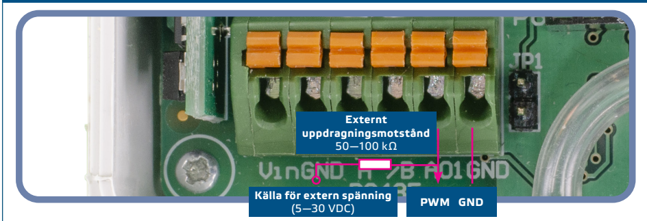
Fig. 6 PWM-anslutning (Öppen kollektor) (JP1 fränkopplad)
