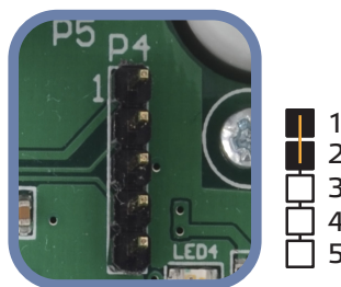
Fig. 10 Återställningsbygel för Modbus holding register
