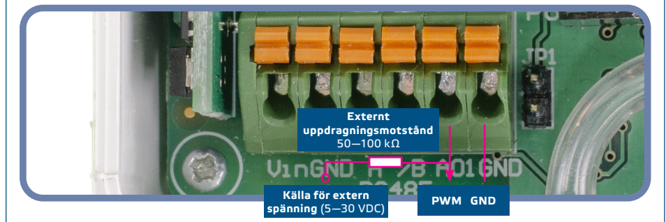
Fig. 6 PWM-anslutning (Öppen kollektor) (JP1 fränkopplat)
