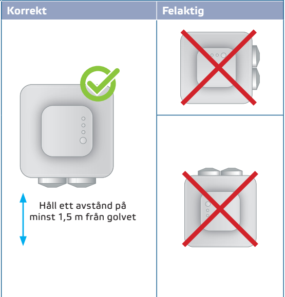
Fig. 5 Monteringsposition
