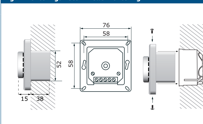
Fig. 2 Monteringsmått - infälld montering
