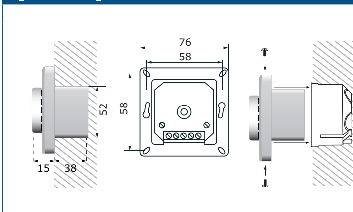
Fig. 2 Monteringsmått
