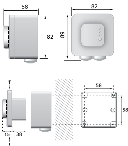
Fig. 4 Monteringsmått – utanaupliggande montering
