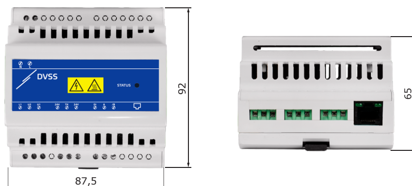
Fig. 1 Monteringsmått
