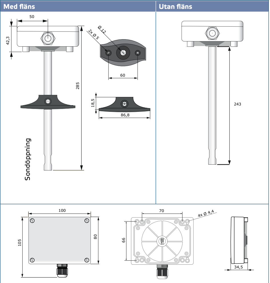
Bild 2 Monteringsposition
