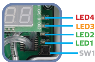
Fig. 8 – Taktomkopplare för sensorkalibrering och återställning av Modbus register - indikeringar
