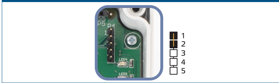
Fig. 10 Återställningsbygel för Modbus holding register
