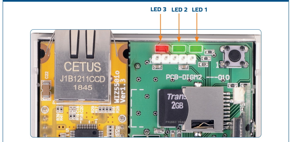
Fig. 6 LED indikeringar
