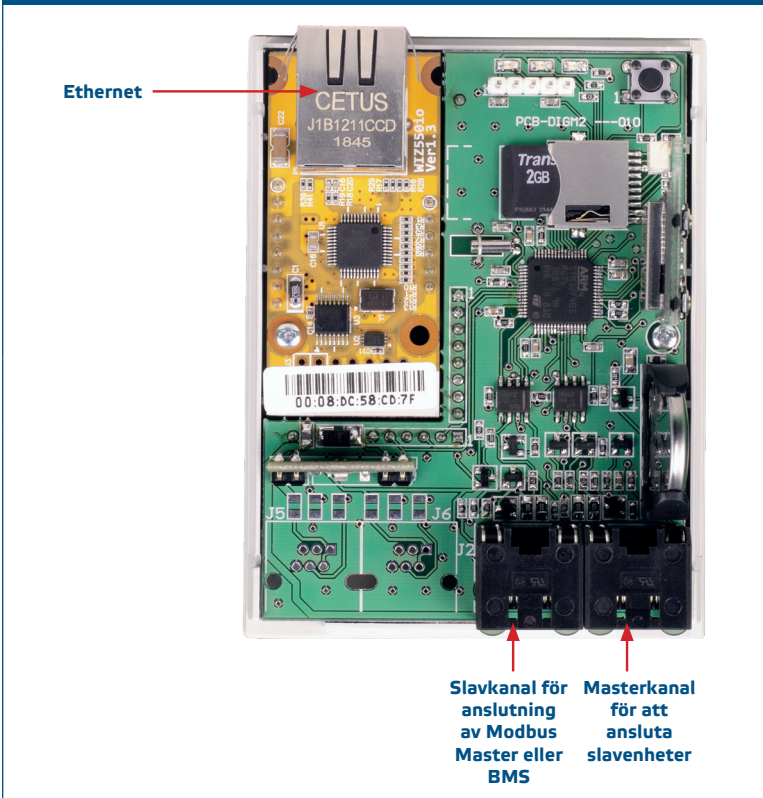
Fig. 3 Koppling
