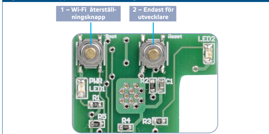
Fig. 5 Taktomkopplare för återställning av Wi-Fi
