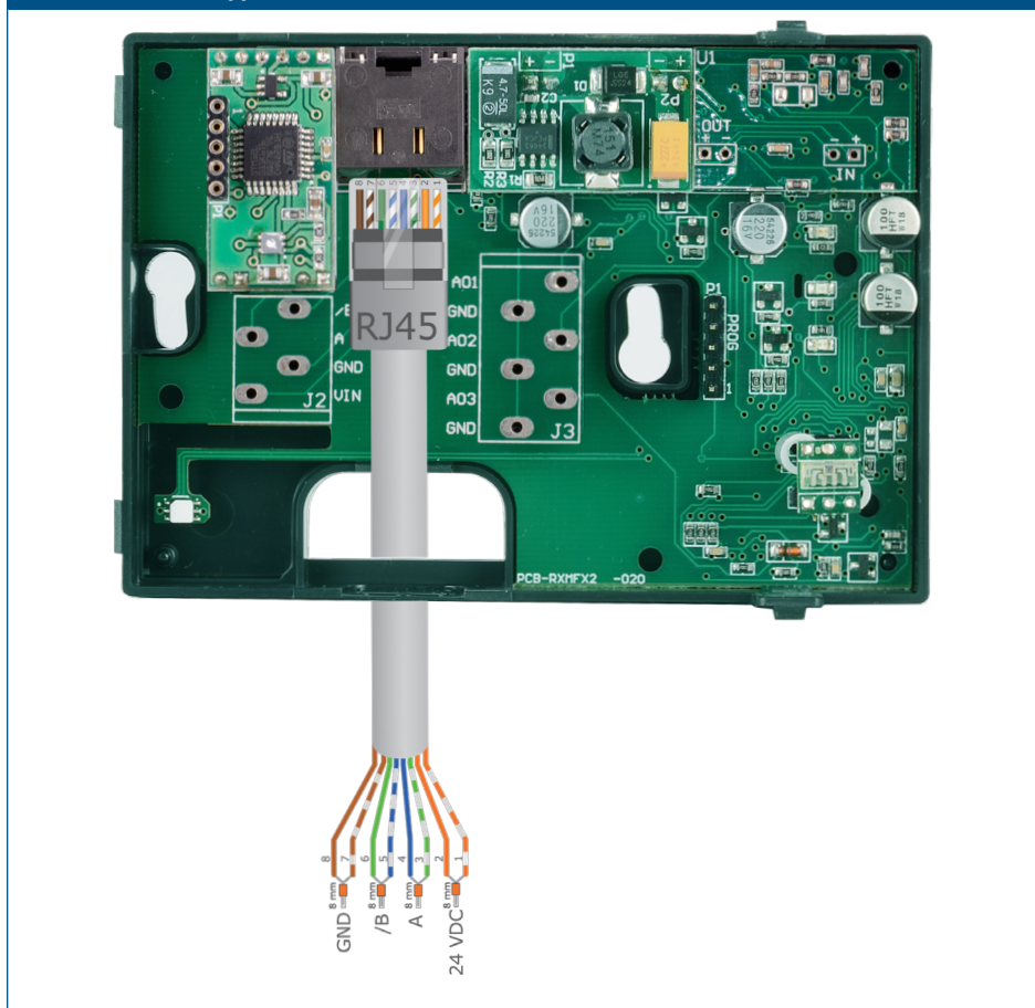
Рис. 4 Схема подключения
