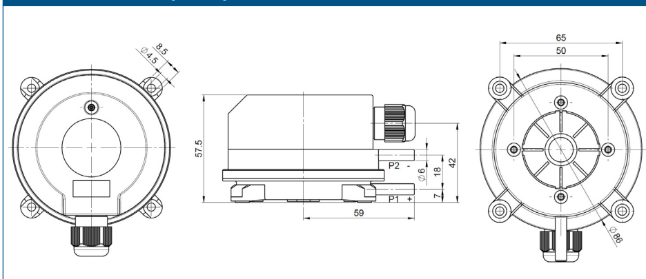
Рис. 2 Монтажные размеры
