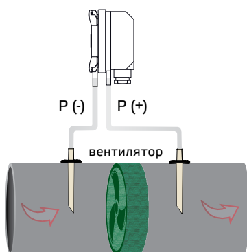
Рис.3.3 Контроль вентилятора
