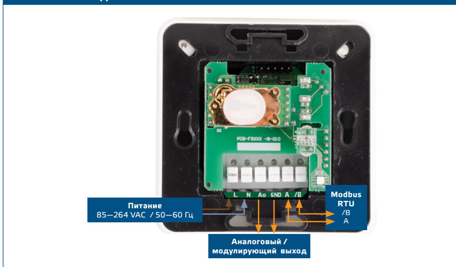
Рис. 1 Схема подключения
