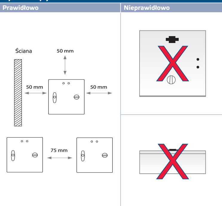
Rys. 2 Pozycja montażowa
