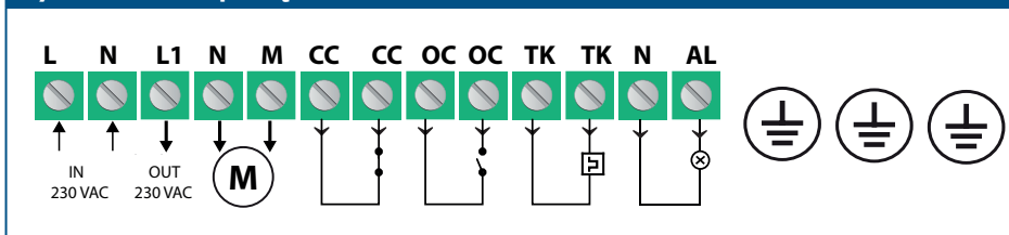
Rys. 3 Schemat podłączenia
