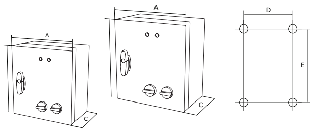
Rys. 1 Wymiary montażowe
