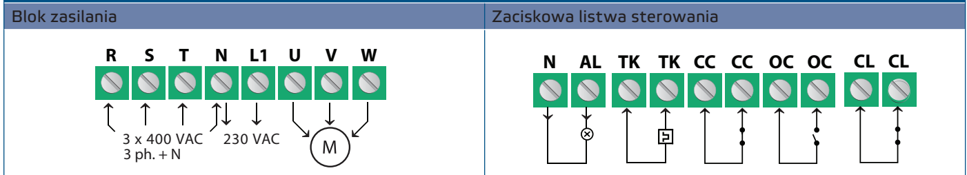
Rys. 3 Schemat podłączenia
