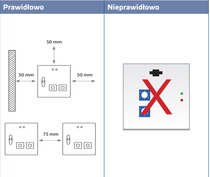
Rys. 2 Pozycja montażowa
