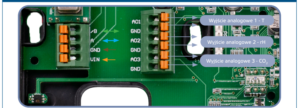
Rys. 4 Schemat podłączenia
