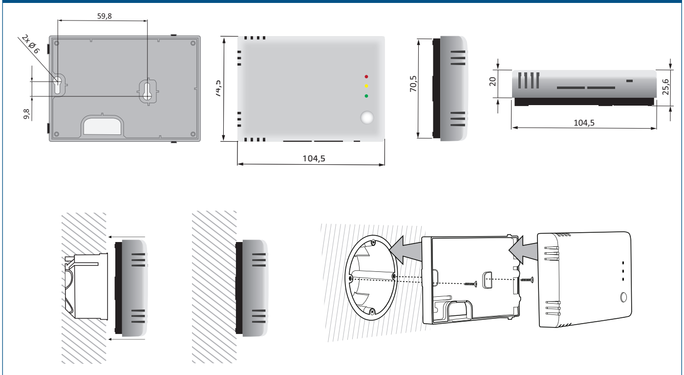
Rys. 2 Wymiary montażowe
