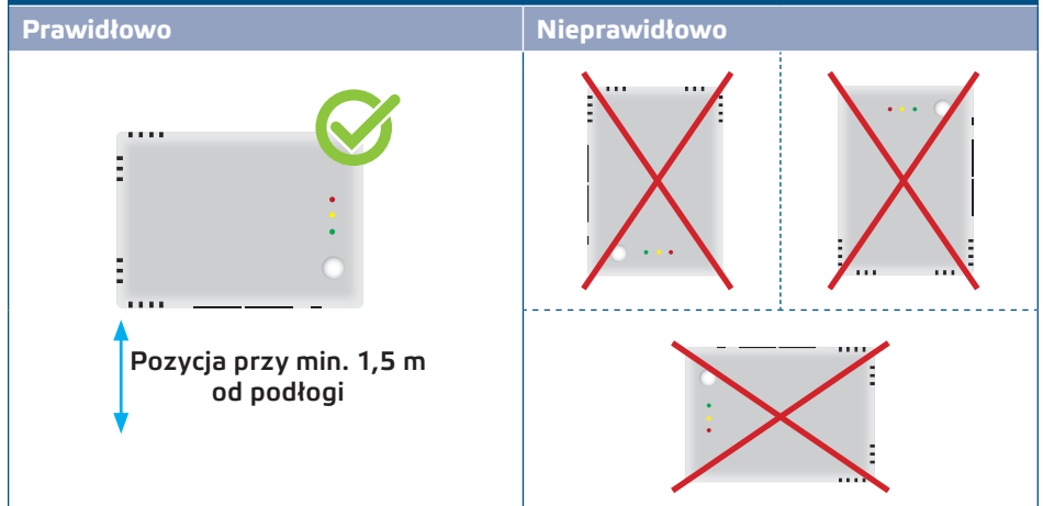
Rys. 3 Pozycja montażowa
