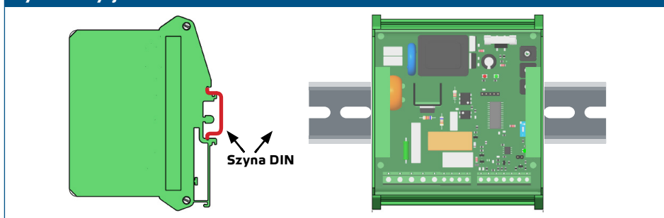
Rys. 2 Pozycja montażowa
