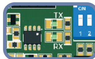
Rys. 8 Wskazanie indykacji komunikacji
