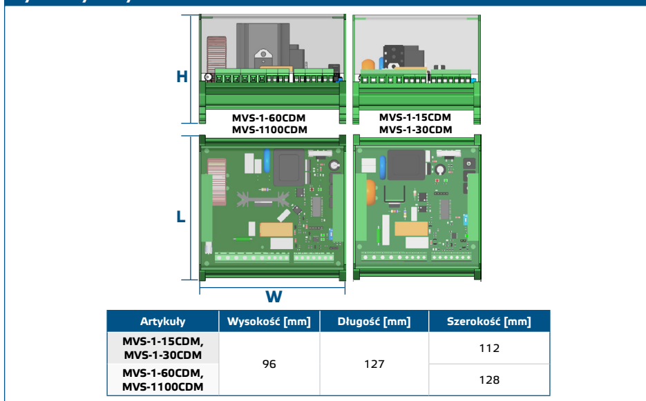
Rys. 1 Wymiary montażowe
