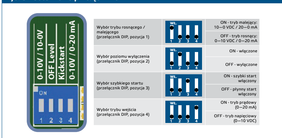
Rys. 3 - Ustawienia przełączników DIP
