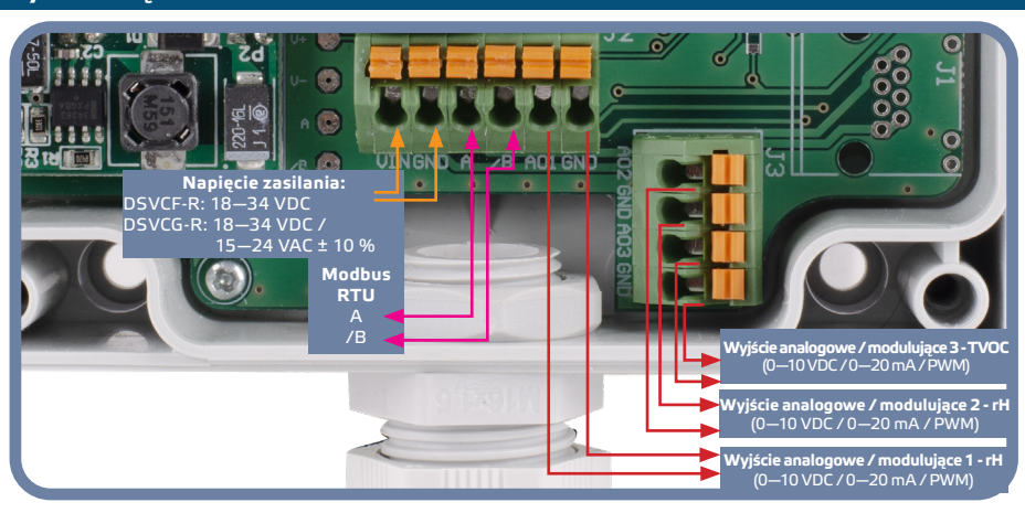
Rys. 4 Połączenia i okablowanie
