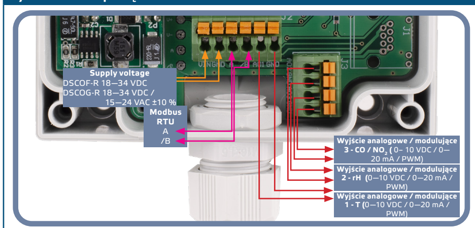
Rys. 4 Schemat podłączenia
