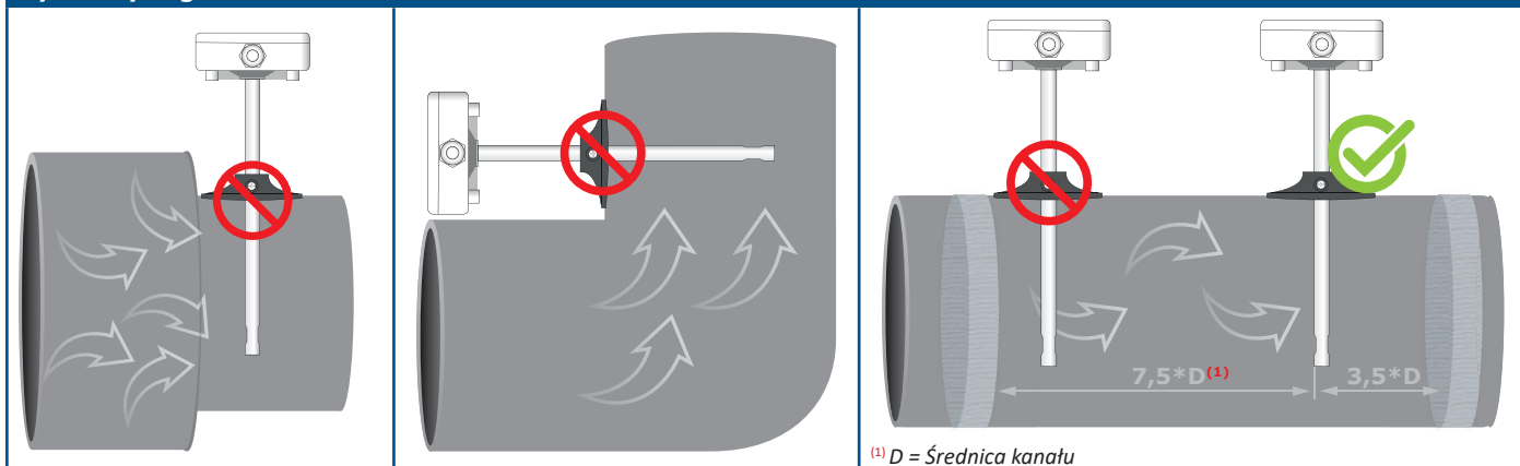
Rys. 3 Wymagania montażowe
