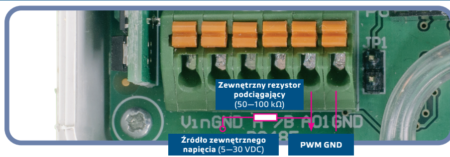
Rys. 6 Połączenie PWM (otwarty kolektor) (JP1 odłączony)
