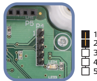
Rys. 10 Zworka resetująca rejestr przytrzymujący Modbus
