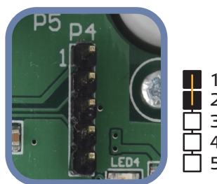
Rys. 8 Zworka resetująca rejestr przytrzymujący Modbus
