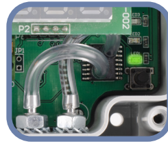
Rys. 5 Sygnalizacja komunikacji Power / Modbus
