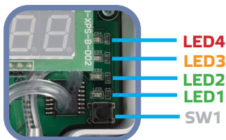
Rys. 6 Kalibracja czujnika i reset rejestru Modbus
