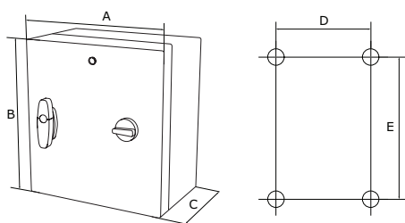
Fig. 1 Bevestigingsafmetingen
