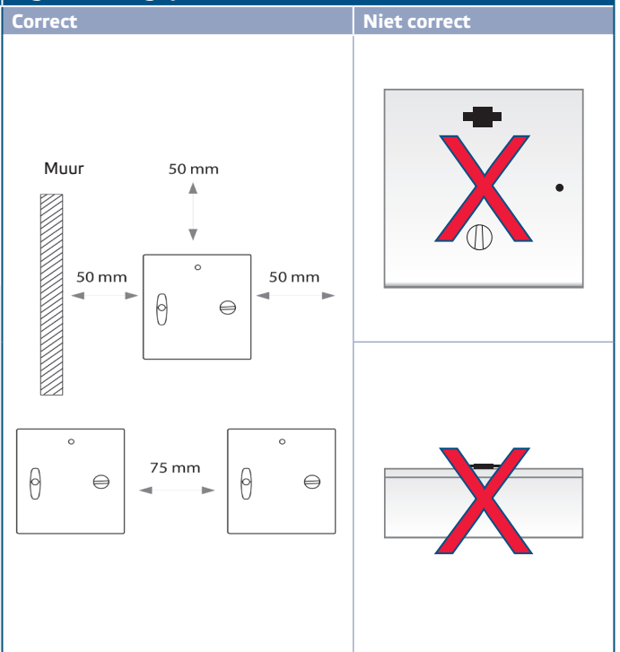
Fig. 2 Montagepositie
