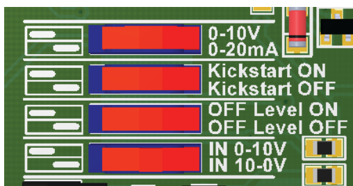
Fig. 4 Microschakelaar posities
