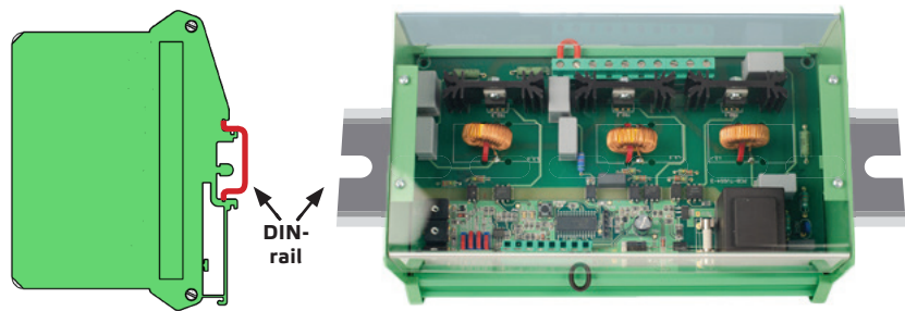
Fig. 2 Montagepositie
