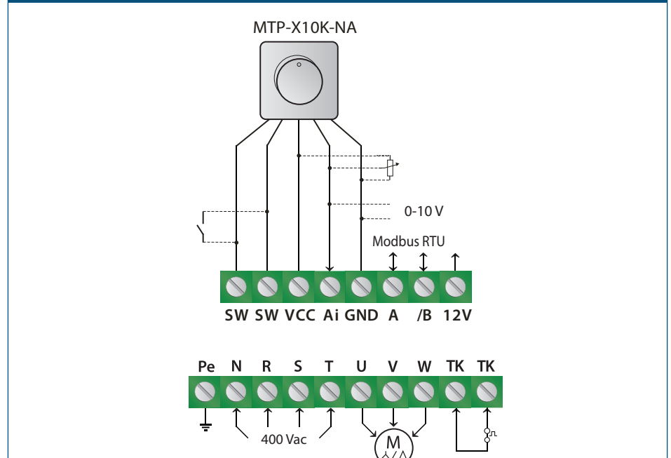
Fig. 3 Aansluitschema
