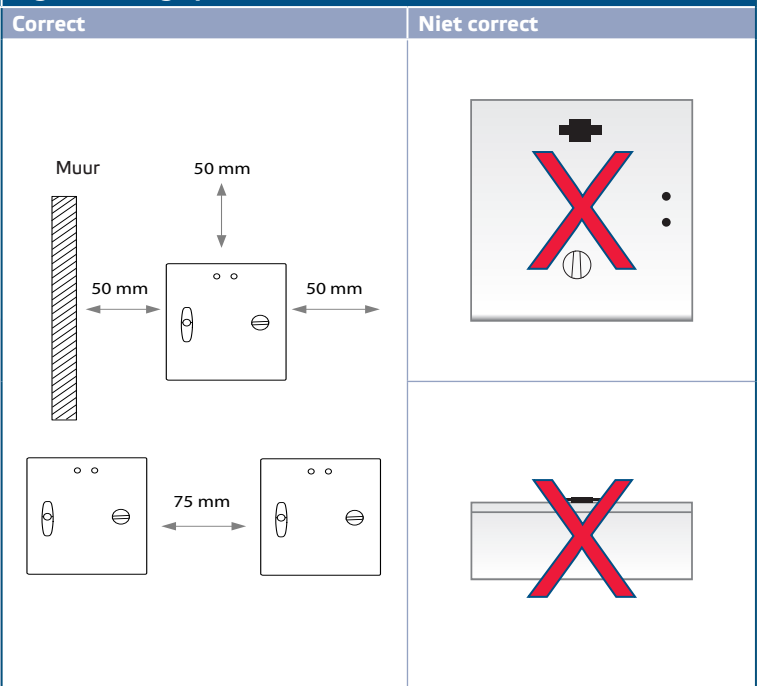
Fig. 2 Montage positie
