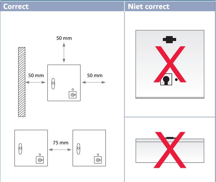
Fig. 2 Montage positie
