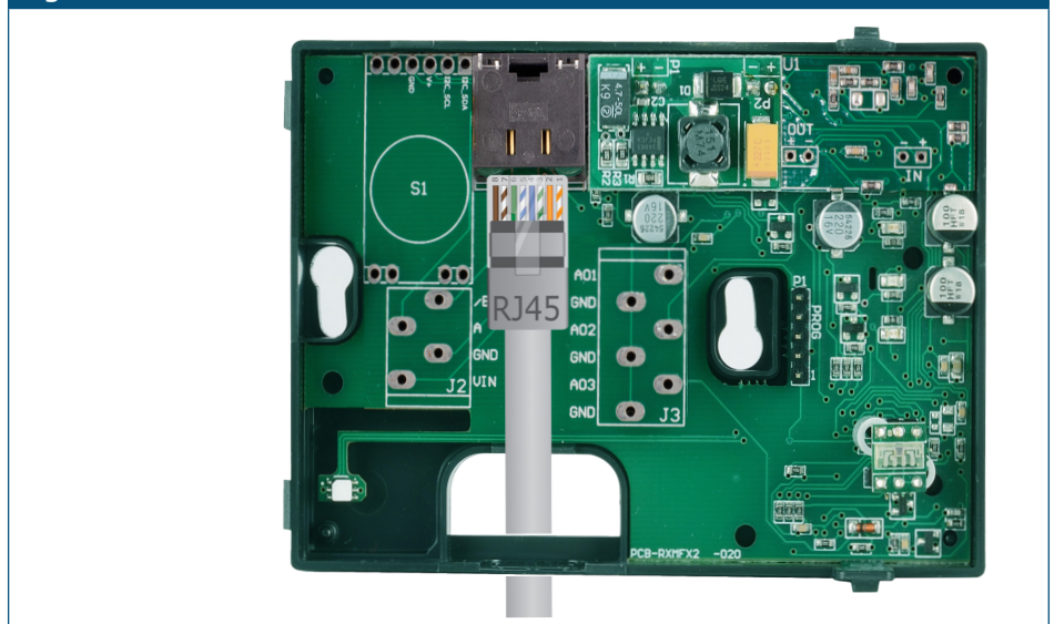
Fig. 4 Aansluitschema
