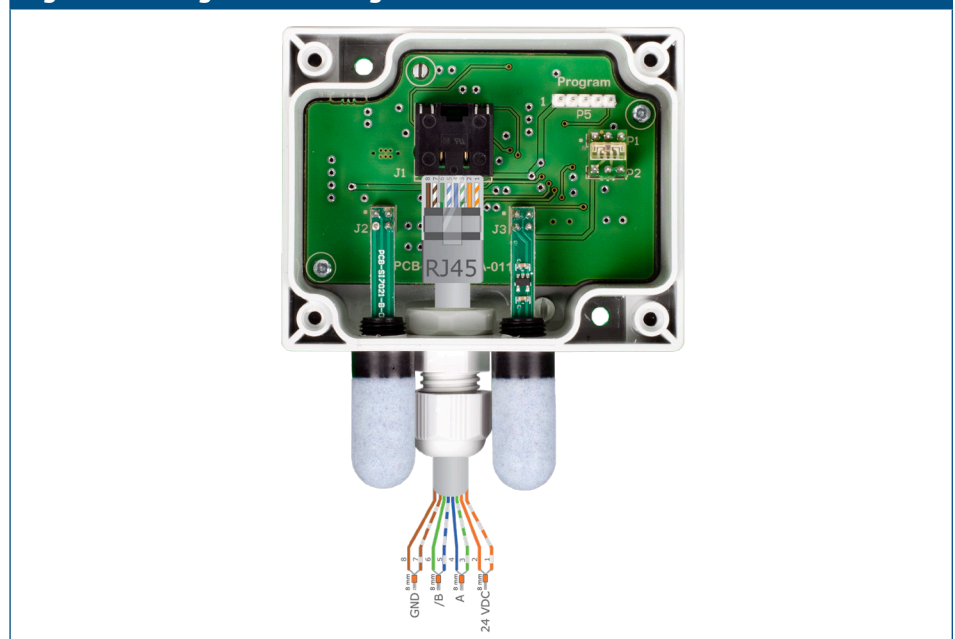
Fig. 4 Bedrading en aansluitingen
