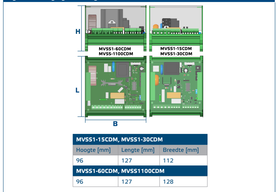
Fig. 1 Bevestiging Afmetingen
