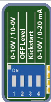
Fig. 4 DIP-schakelaar instelling
