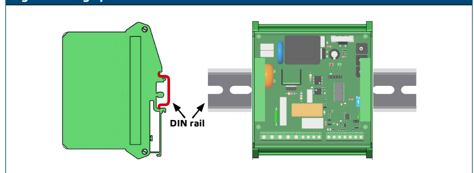
Fig. 2 Montage positie
