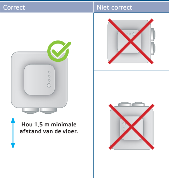
Fig. 5 Montagepositie
