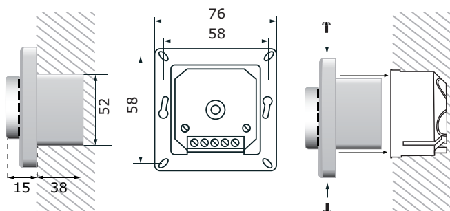
Fig. 2 Afmetingen - inbouw
