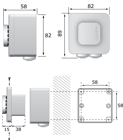
Fig. 4 Afmetingen - opbouw montage
