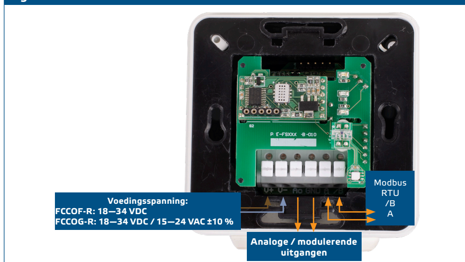
Fig.1 Aansluitschema
